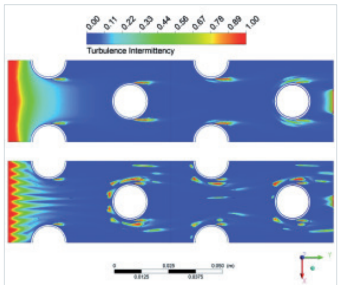
Bild 12 Turbulenzgrade im Vergleich zur flachen Lamelle (oben)
