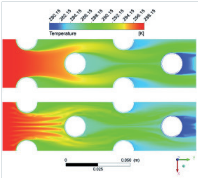
Bild 9 Lufttemperaturprofile im Vergleich zur flachen Lamelle (oben)
