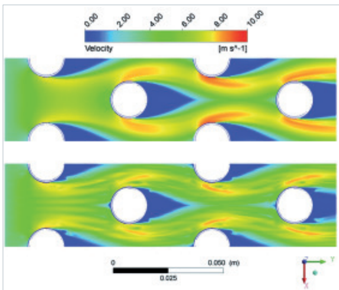
Bild 11 Geschwindigkeitsprofile im Vergleich zur flachen Lamelle (oben) 3)
