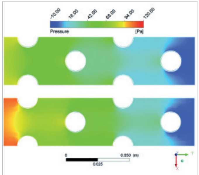
Bild 10 Druckverläufe im Vergleich zur flachen Lamelle (oben)
